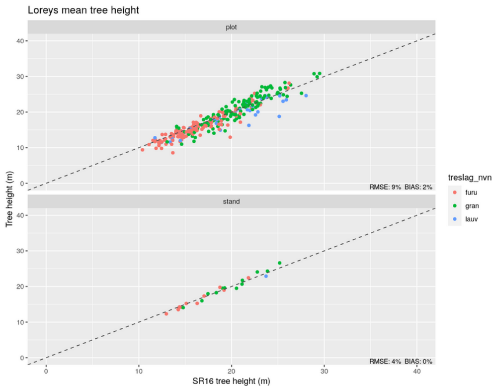
Figur 5: Sammenligning av middelhøyde fra feltmålinger og SR16 i Asker. Plot = flåte, stand = bestand.
