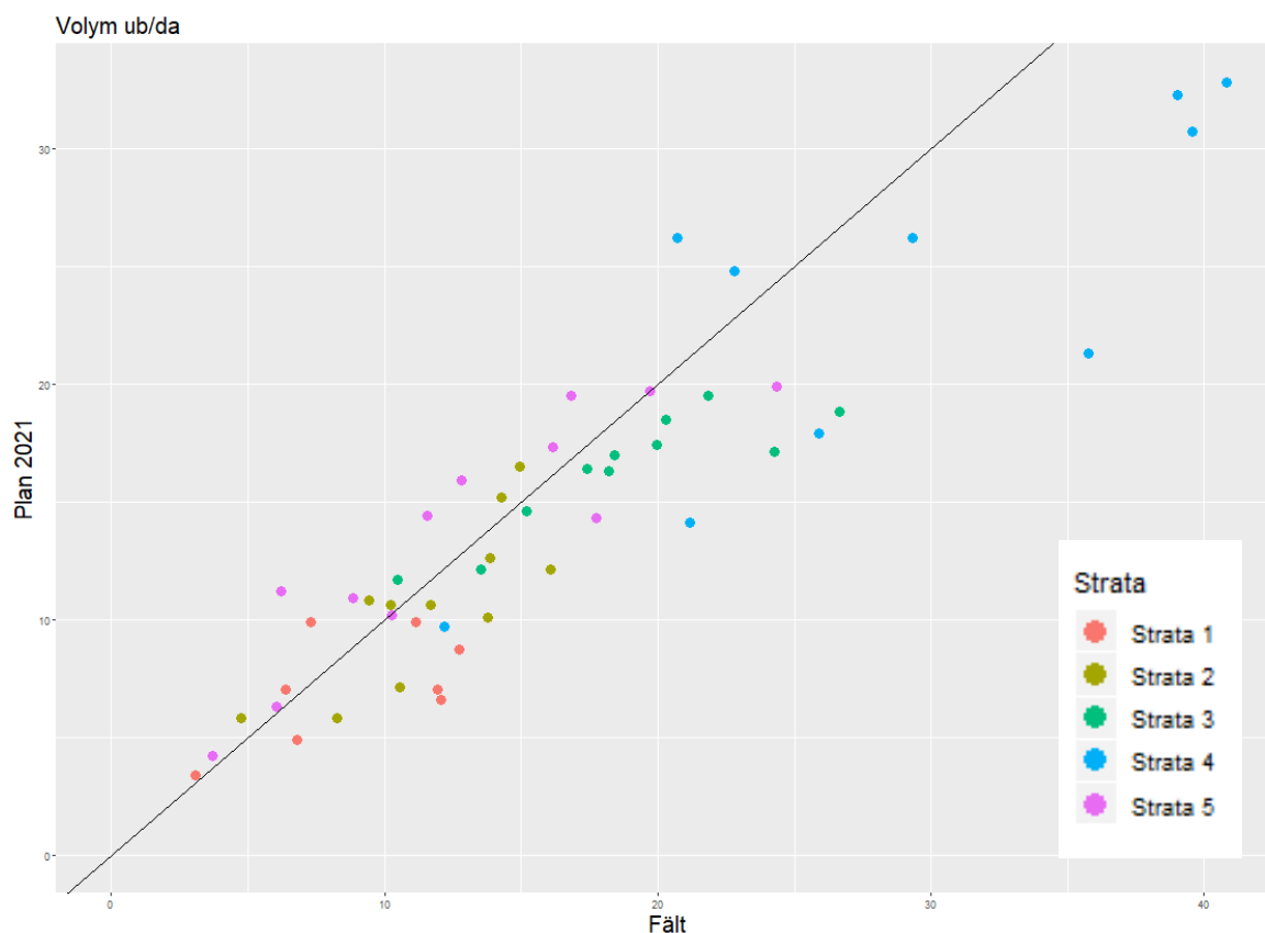
Figur 30. Sammenligning av volum fra feltmålinger og SR16 i Namdal. Hvert punkt er ett bestand. Feltemålte verdier på horisontal akse («Fält») og SR16 på vertikal akse («Plan 2021»). Farge angir stratum (1 = gran høyde 8-11m, 2 = gran høyde 11-13m, 3 = gran høyde 13-16m, 4 = gran høyde >16m, 5 = furu høyde >8m).
