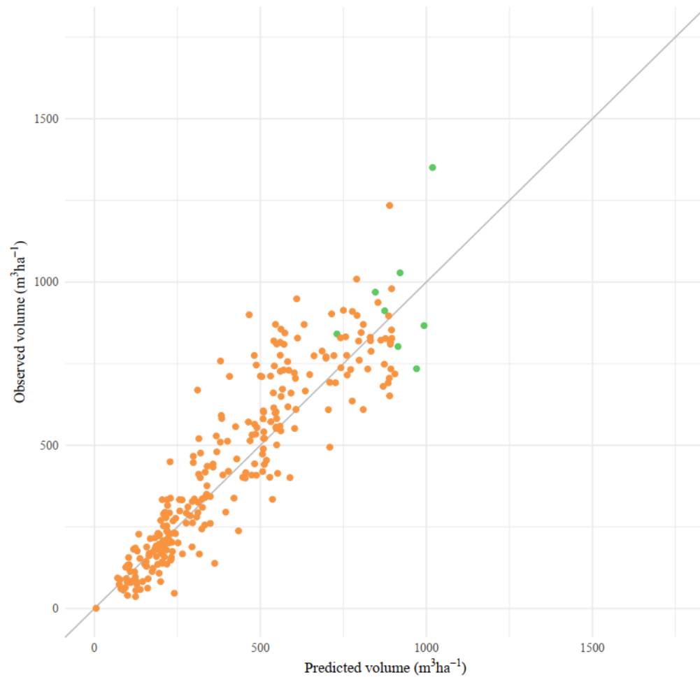
Figur 26: Eksempel for ekstrapolasjon av egenskaper med regresjonsmodeller (grønne punkter) der kNN ikke kan anvendes.
