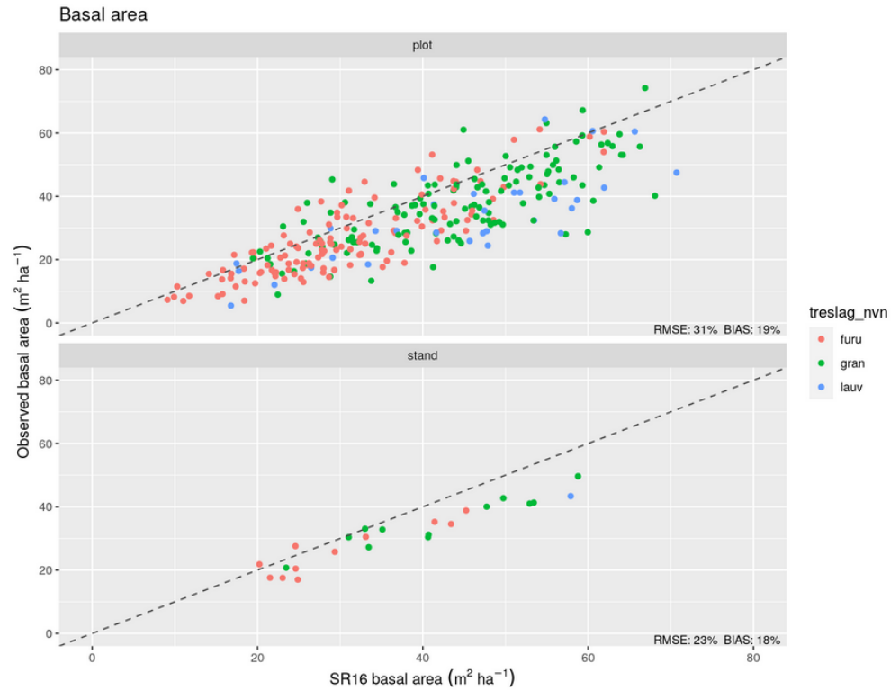
Figur 4: Sammenligning av grunnflate fra feltmålinger og SR16 i Asker. Plot = flåte, stand = bestand.
