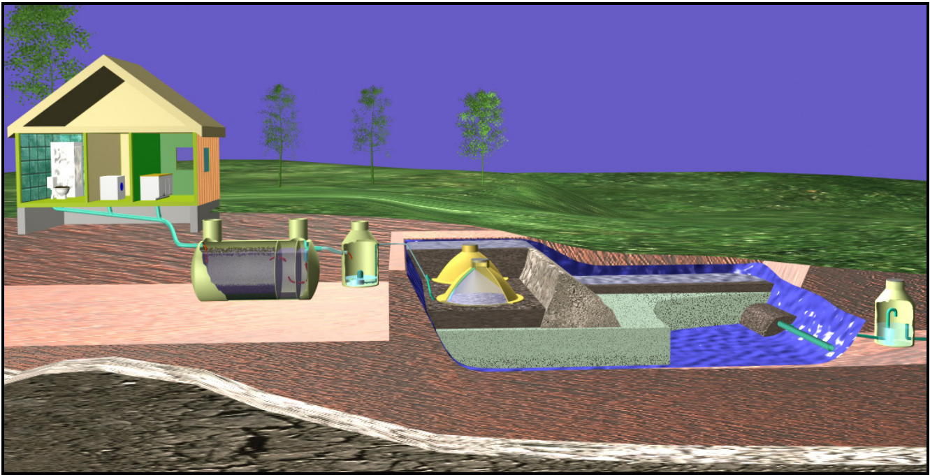
Figur 4. Prinsippskisse av filterbedanlegg med slamavskiller, pumpekum, biofilter, filterbasseng og utløpskum.
