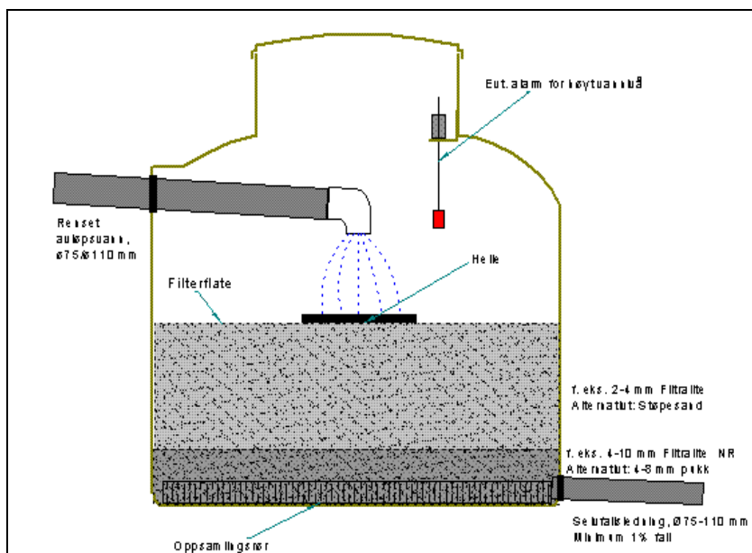
Figur 15. Eksempel på partikkelfjerningsfilter før rensert avløpsvann fra minirensanlegg føres til infiltrasjon.
