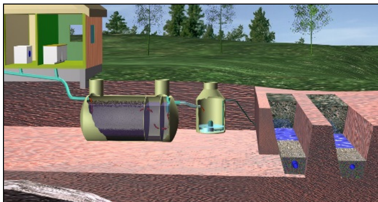
Figur 12. Prinsippskisse av grunt infiltrasjonsanlegg. Vannet renner fra hus til slamavskiller og videre til pumpekum før støtbelastning ut i infiltrasjonsgrøfter etablert i stedlige masser.
