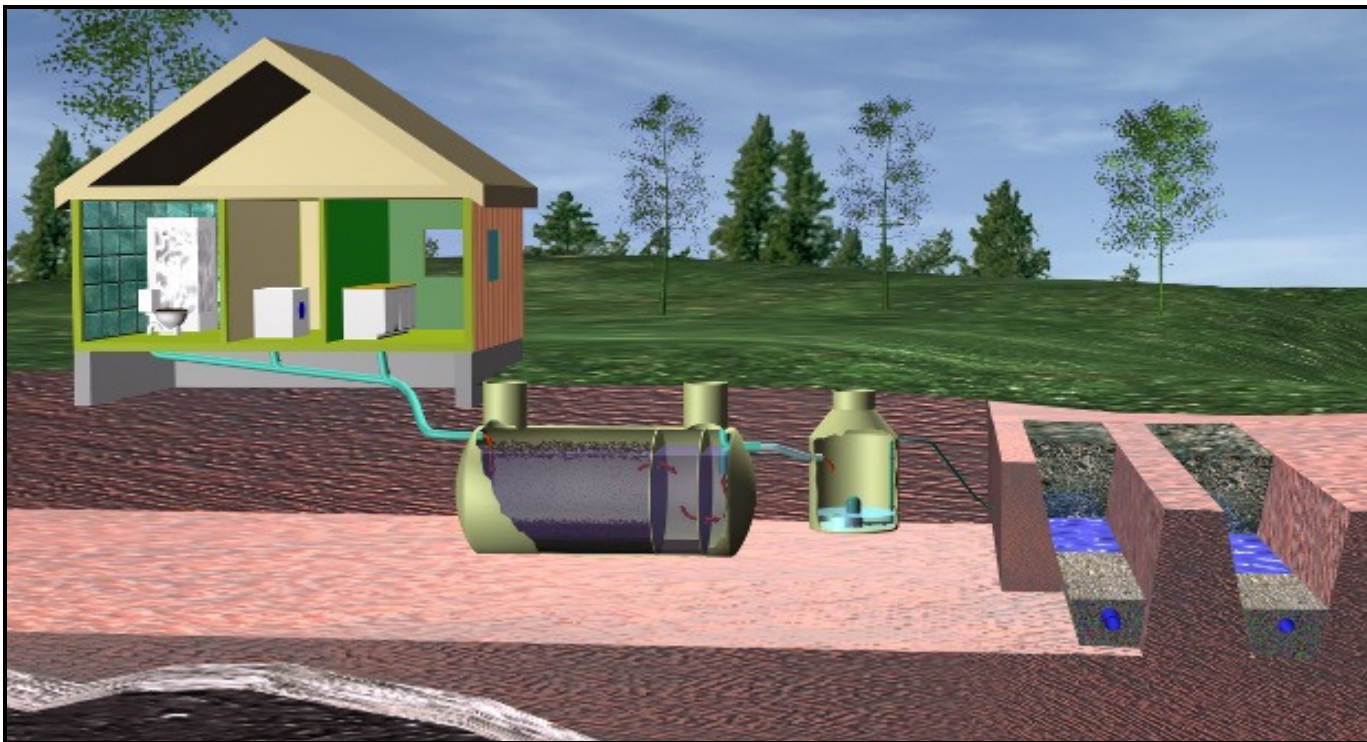
Figur 2. Prinsskisse av grunt infiltrasjonsanlegg. Vannet renner fra hus til slamavskiller og videre til pumpekum før støtbelastning ut i infiltrasjonsgrøfter etablert i stedlige masser.
