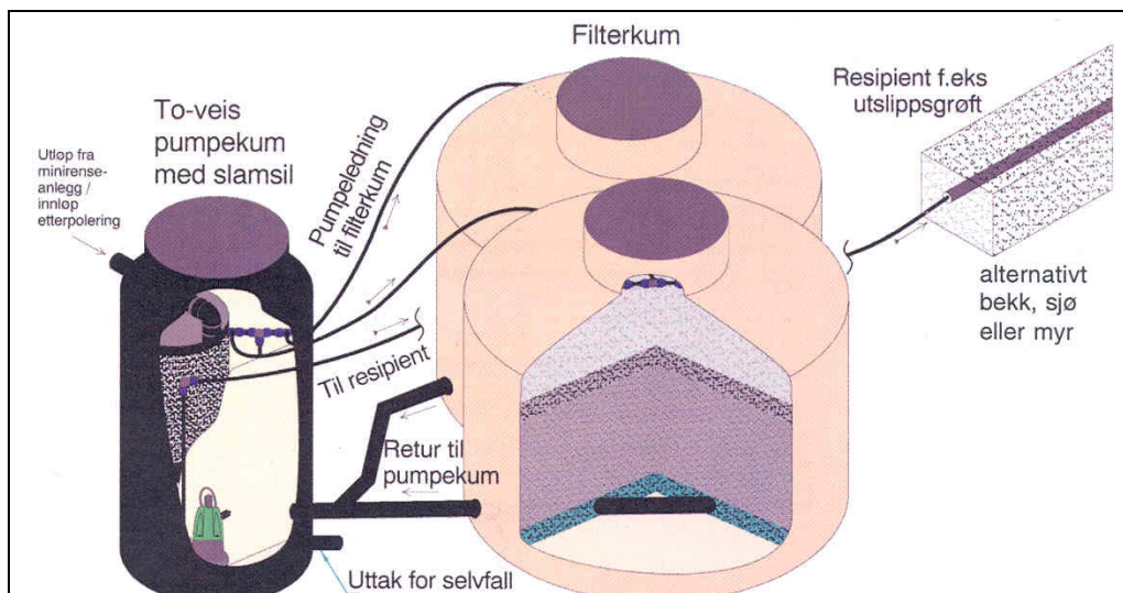
Figur 16. Eksempel på etterrenningsanlegg med biofilter før rensert avløpsvann fra minirensanlegg føres til infiltrasjon.
