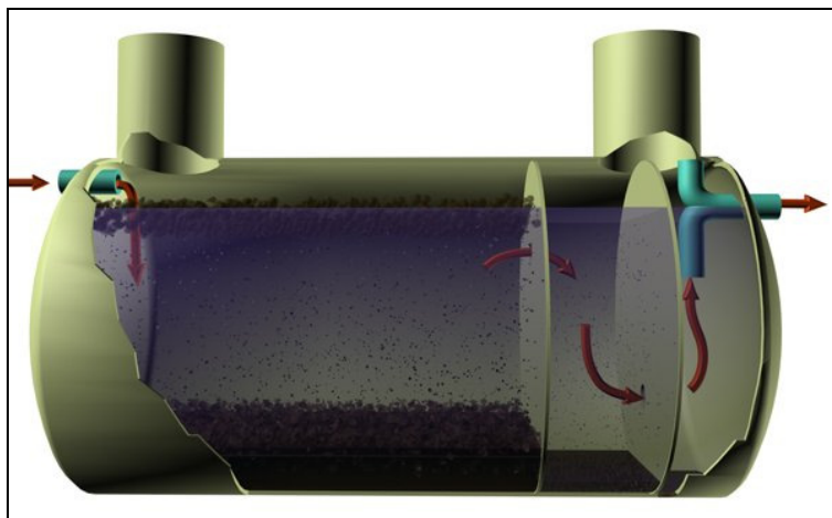
Figur 21. Prinsippskisse av trekamret slamavskiller som viser vannets strømningsvei gjennom kummen.
