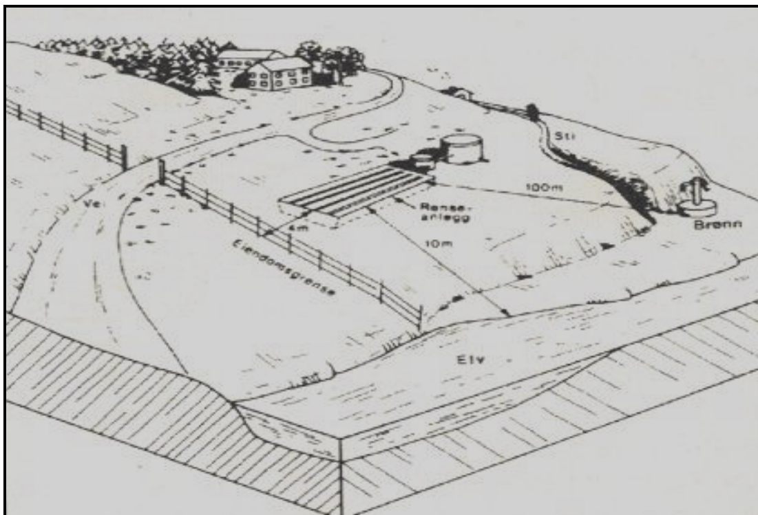
Figur 1. Eksempel på hensiktsmessig plassering av et infiltrasjonsanlegg i forhold til vannuttak, elv, eiendomsgrense og sti. (Tilsvarende er det nødvendig å planlegge utslipp av rensed avløpsvann til grunnen.) Ved utslipp til elv, sjø eller ferskvann bør det også vurderes om utslippet kan få uheldige virkninger på miljøet.
