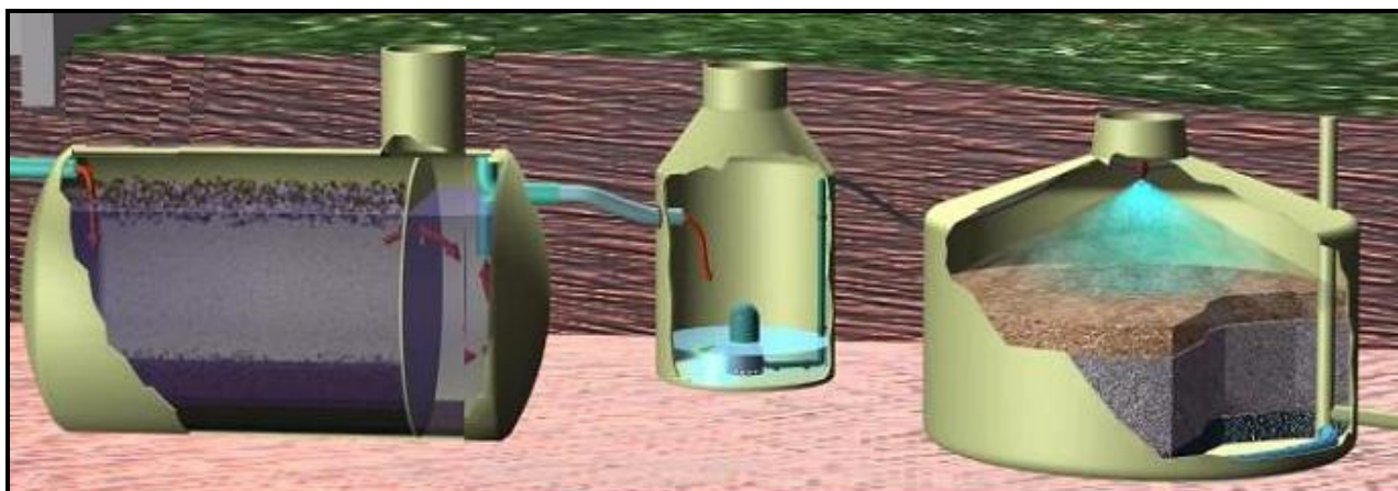
Figur 6. Prinsippkisse av et gråvannsrenseanlegg med slamavskiller, pumpekum og biofilter. Renset vann ledes til etterrensing i stedlige masser eller i lukket rør til et sted med overflatevann.
