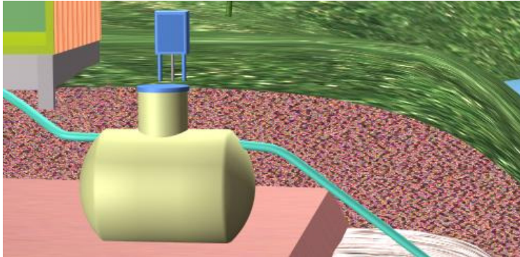
Figur 14. Prinsippskisse av minirenseanlegg. Vannet renner fra bolig til minirenseanlegget som i de fleste tilfeller består av en tank. Renseprosessene skjer via flere rensetrinn gjennom tanken og rensset vann ledes i lukket rør til overflateresipient, drensssystem eller løsmasser.
