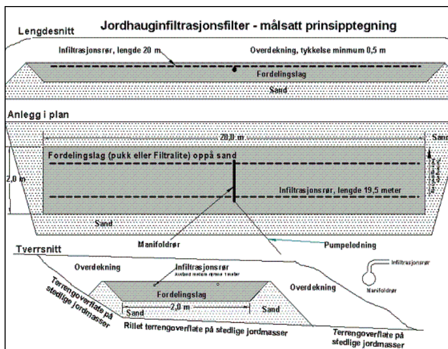
Figur 13. Eksempel på målsatt prinsipptegning av prosjektert jordhauginfiltrasjonsanlegg
