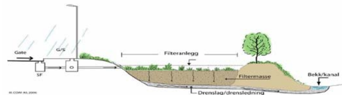
Prinsippskisse av et rensfilter etablert inn i grønnstruktur. Fra rapport UTB 2007/2 på http://www.vegvesen.no .
