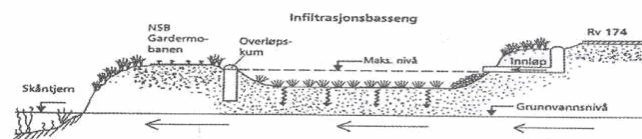
Infiltrasjonsbasseng for overvann fra veg på Rv35 ved avkjøring til Oslo Lufthavn. Fra håndbok 261 på http://www.vegvesen.no .
