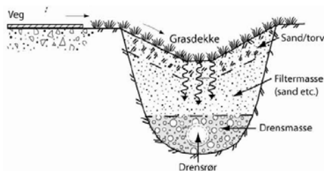
Filtergrøft med filtermaterialer for optak og nedbryting av forurensning. Fra Rapport UTB 2007/2 på http://www.vegvesen.no
