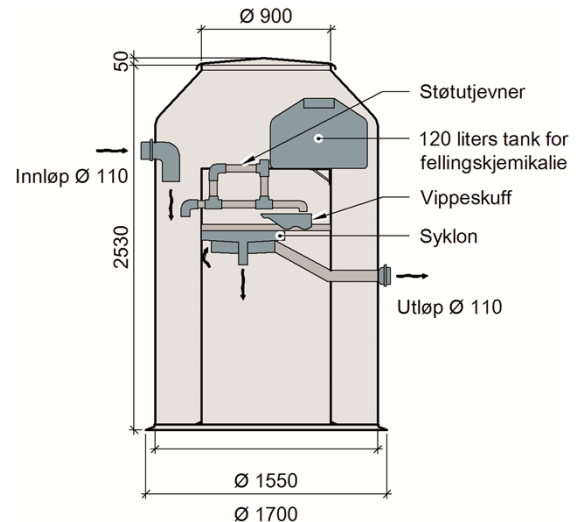
Fig. 1 Wallax W1 minirensesanlegg
